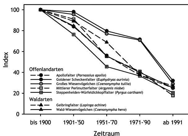
Abb. 2: Arealentwicklung von Tagfalterarten des Offenlandes und der Wälder auf Basis von Messischblättern in Deutschland. 100 = alle jemals besiedelten MTB (aus FARTMANN et al. 2019).
